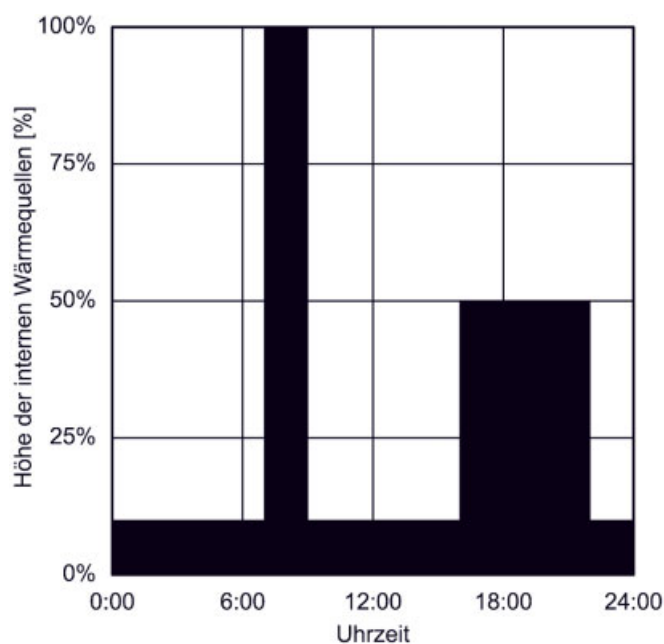
Bild 16. Tägliches Lastprofil der internen Wärmequellen Fig. 16. Daily load profile of the internal heat sources
