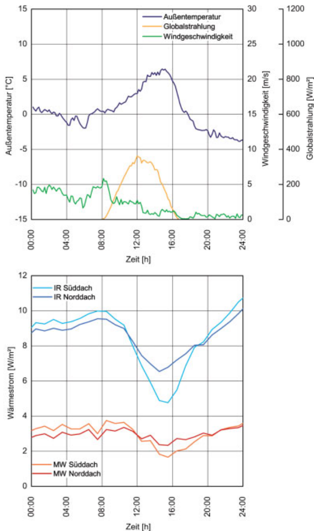
Bild 9. Wetterbedingungen und Wärmeströme an einem strahlungsreichen Tag (8. Januar 2008)
