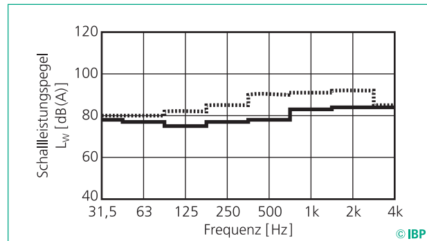
Bild 5: A-bewertete Schalleistungspegel der Schornsteinmündung: gemessene Werte (durchgezogene Linie) und Garantiewerte (gestrichelte Linie).
